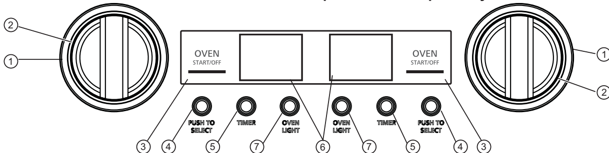
Panel de Control del Horno de 48" para Hornos Izquierdo y Derecho
