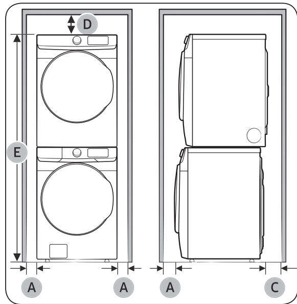
Instalación apilada
