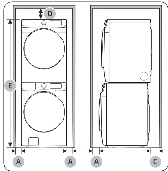
Installation superposée
