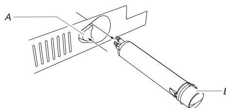
A. Boutons d'éjection B. Bouchon du filtre
