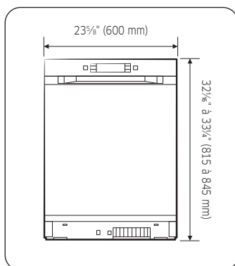
Vue avant
