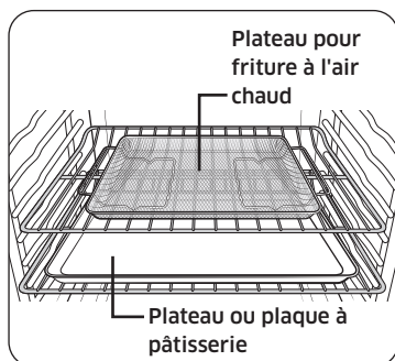
Emplacement recommandé pour le plateau pour friture à l'air chaud
