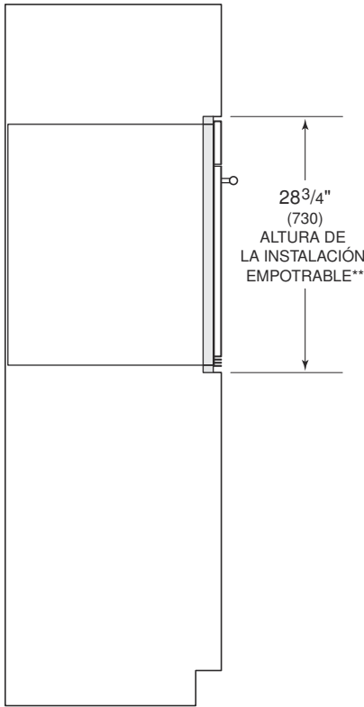
VISTA LATERAL
