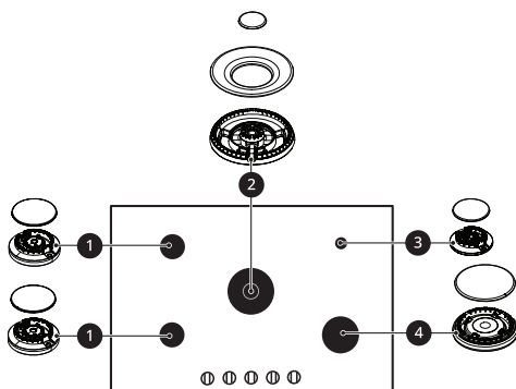
1 Tête et capuchon du brûleur moyen
