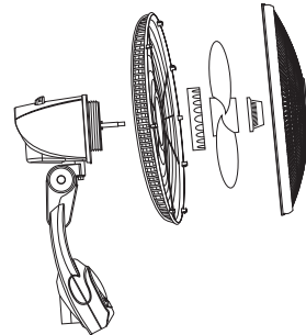
1. Assemble Fan Head
